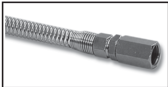
Raccordo per spirale fil. femmina "girevole" Female connection for spiral hose with spring "swivelling"
